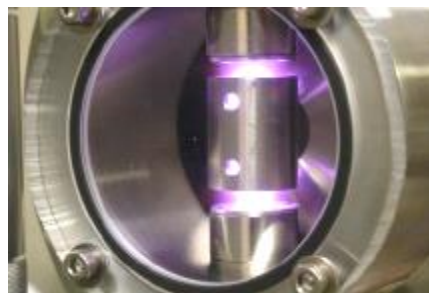
都市大加速器 PIGイオン源
